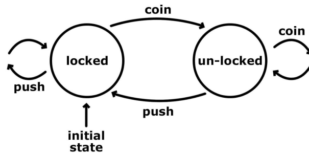
Figura 2.1: Ilustración de una máquina de estados finitos
